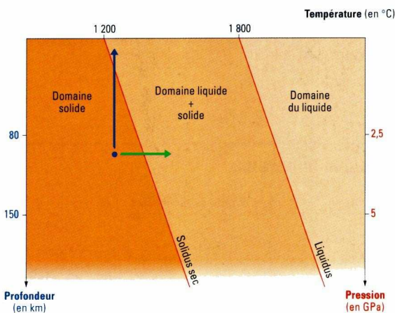
Courbe de fusion des péridotites non hydratées (anhydres).
