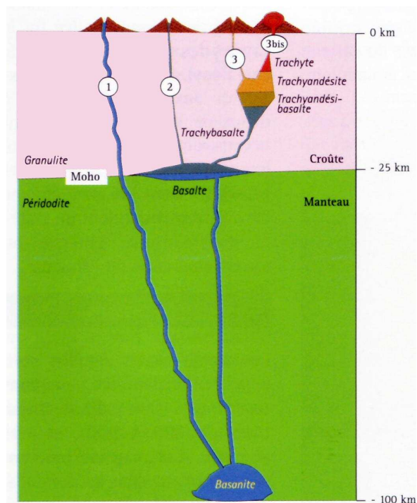
Les 3 possibilités de transit des magmas dans la Chaîne des Puys (d'après Alain de Goër et Pierre Lavina, 1999).
