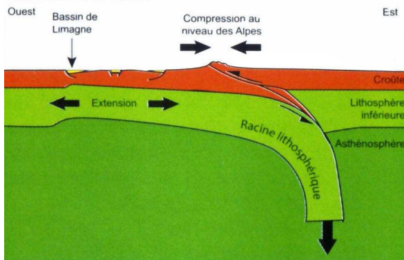
1. Enfoncement de la racine lithosphérique par subduction et création de bassins sédimentaires lors de l'extension
