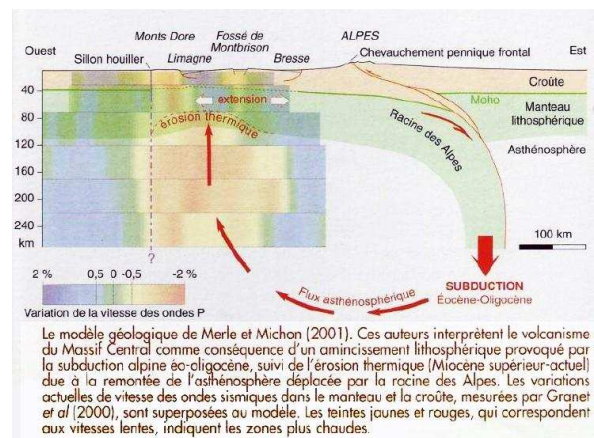
Synthèse en un seul schéma
