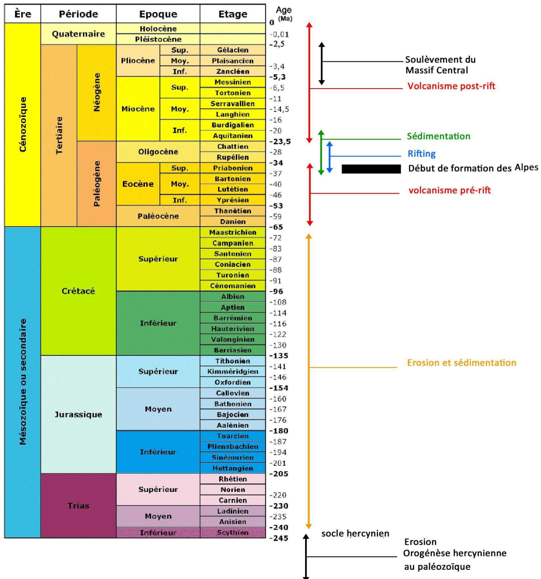
Chronologie de quelques événements géologiques affectant le Massif Central
