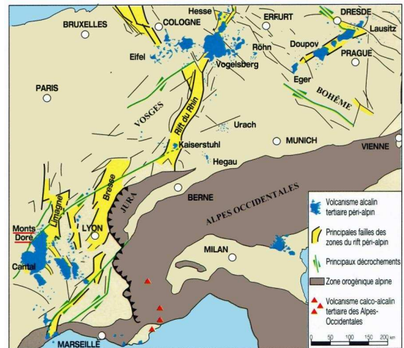
Carte des principales provinces volcaniques cénozoïques d'Europe de l'Ouest en relation avec les bassins sédimentaires péri-alpins (zones de rift)
