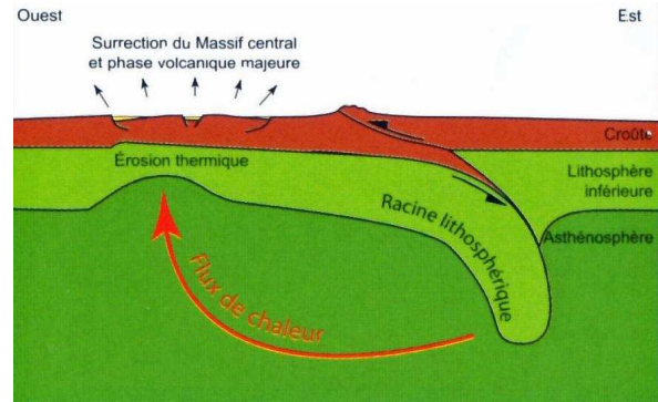
2. Le flux de chaleur amincit la partie basale de la lithosphère par « érosion thermique » et s'ensuit une surrection du Massif Central.
